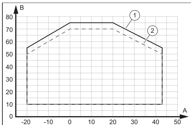
A Offset vanj. tem 1 Granice primjene, normalni pogon WW B Temperatura ogrjevnice vode 2 Granice primjene, startna faza WW
