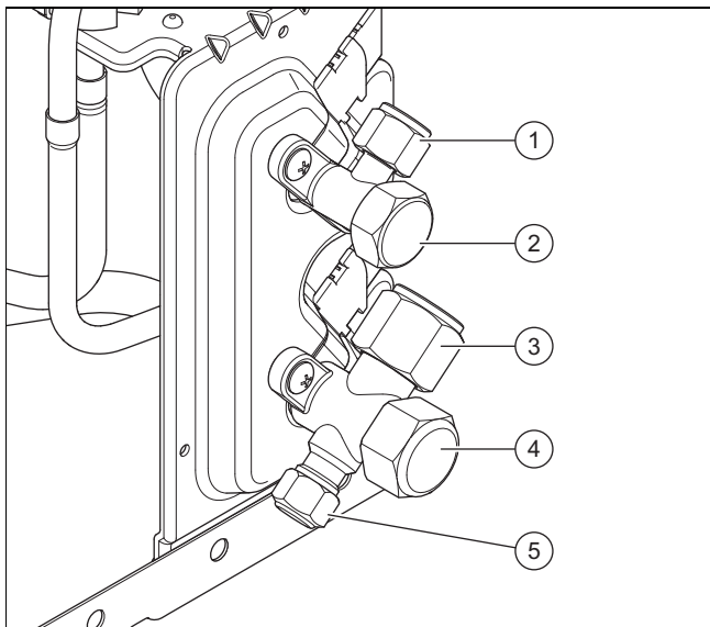
1 Priključak za vodu za tečnost 4 Zaporni ventil za vodu za vreli gas 2 Zaporni ventil za vodu za tečnost 5 Priključak za održavanje sa šreder ventilom 3 Priključak za vodu za vreli gas
