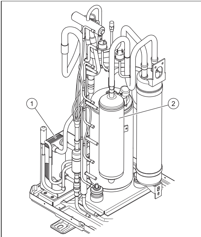
1 Među izmenjivač toplote 2 Separator rashladnog sredstva
