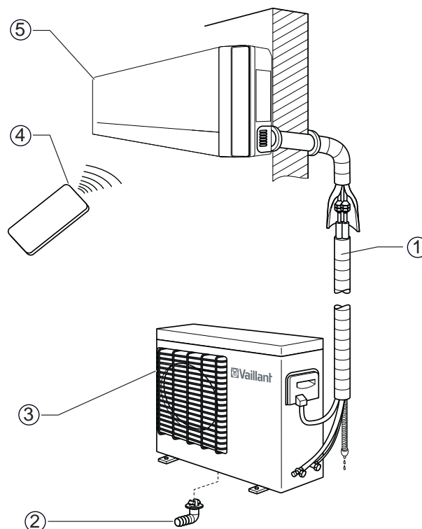
Slika 5.1 Komponente jedinice
